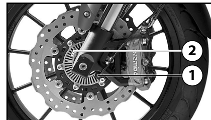
1. Capteur de roue avant 2. Rotor de capteur avant
